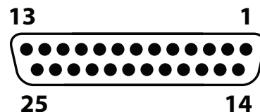
Apollo 16 DB25メスコネクターピン配列
