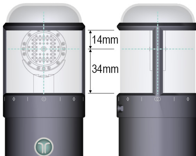
図4-4 Sphereマイクロフォンと Neumann U67/87(左)、AKG 414(右)のダイアフラムの位置
