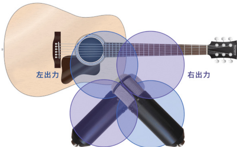
図7-6 ブルムラインテクニックを用いたステレオギター収録
